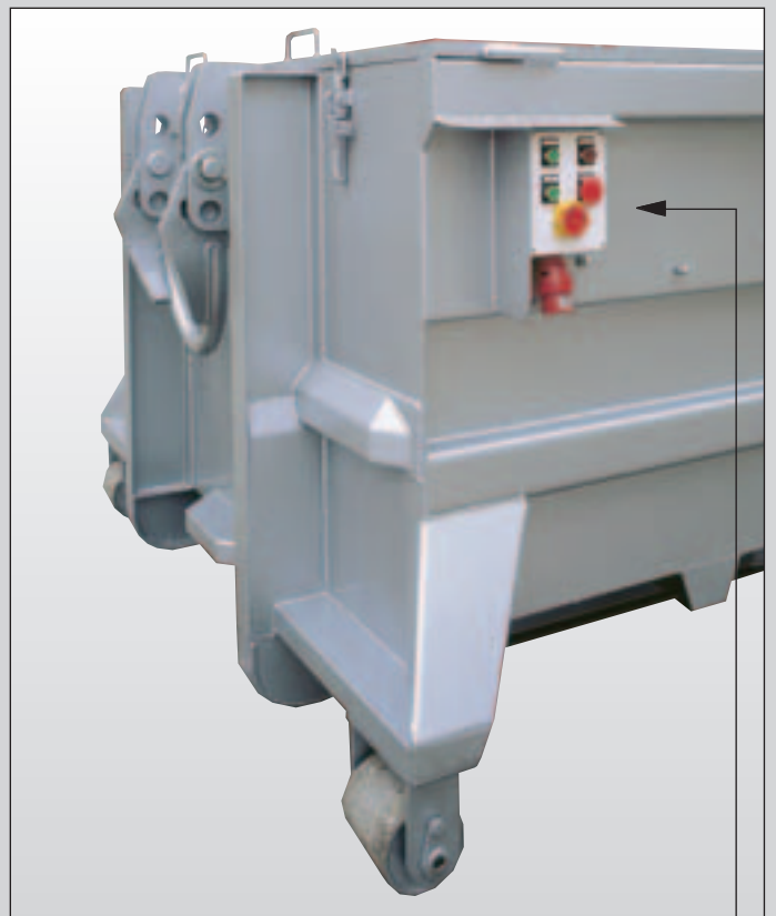
Das Steuerpanel ist übersichtlich und komplett. Controlpanels for easy handling, including all safety-switches.
