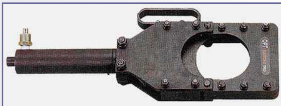
HT-100 Schneidkapazität bis 100 mm Ø Aussendurchmesser
